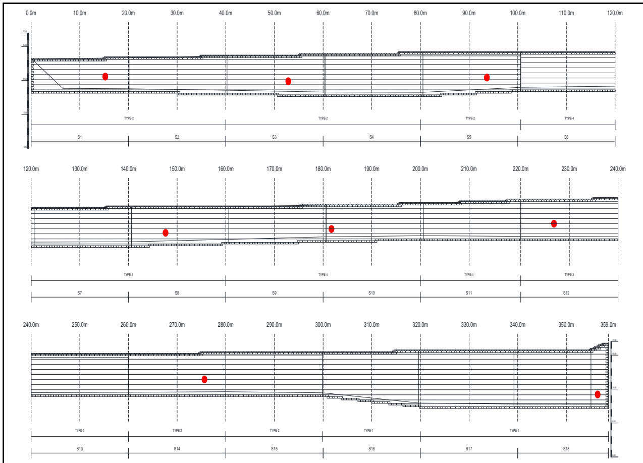
【그림 4.9】 옹벽 조사 분할구간
