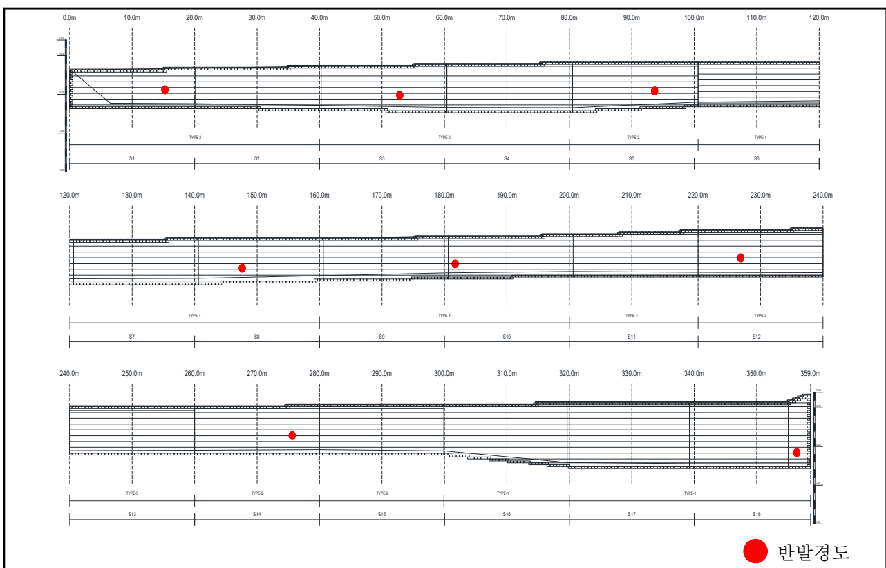
【그림 4.11】 재료시험 위치도
